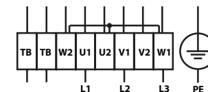
Y- 400 В, 3ф.
