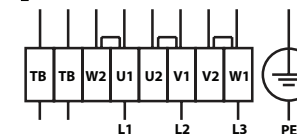
Схема 2 Δ- 230 В, 3ф.
